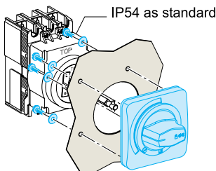
EZC100/125
