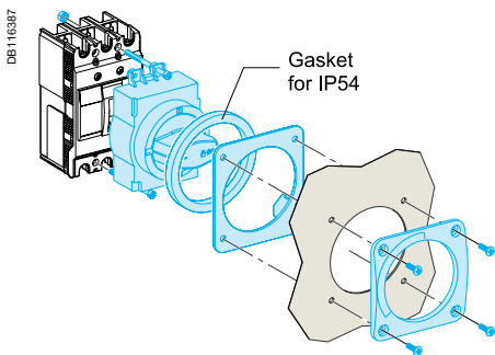
EZC100/125
