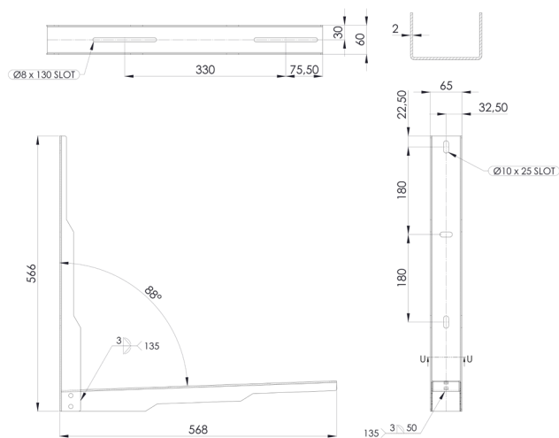
ACB.W01.600 30000 - 60000 BTU
