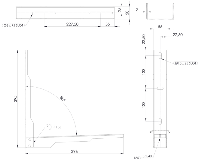
ACB.W01.600 30000 - 60000 BTU
